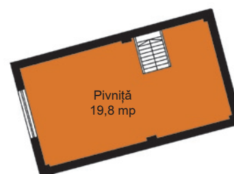
PLAN DEMISOL
