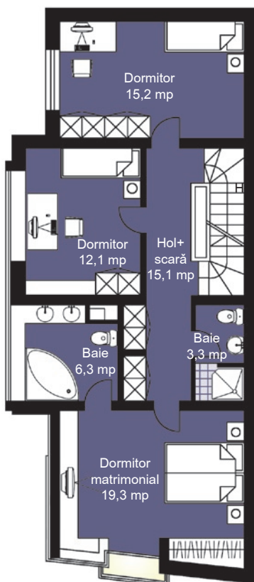
PLAN ETAJ
